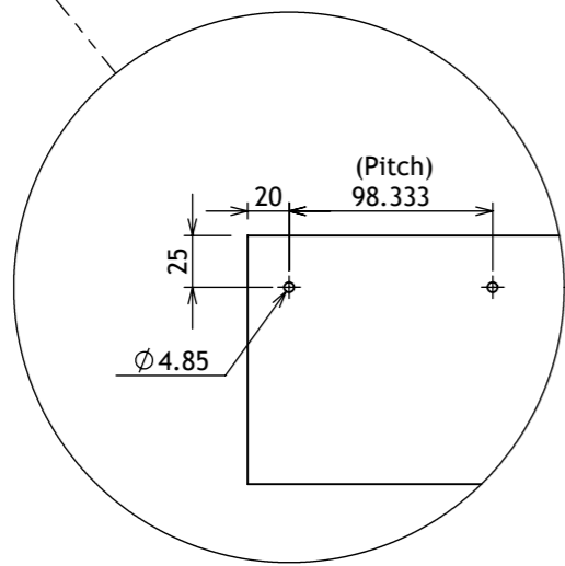
D (1 : 4)
